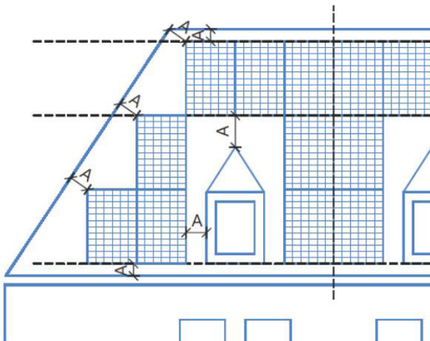
Abbildung 56: Grundordnung der Solaranlagen bei geneigten Dächern
