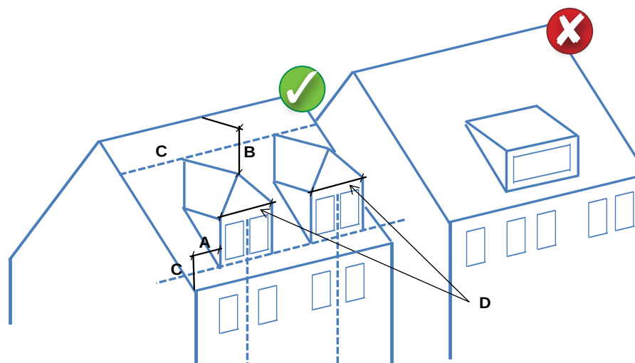
Abbildung 55: Anordnung der Dachaufbauten unter Berücksichtigung der Fassadengliederung und Einhaltung der Mindestabstände und Größenvorgaben
