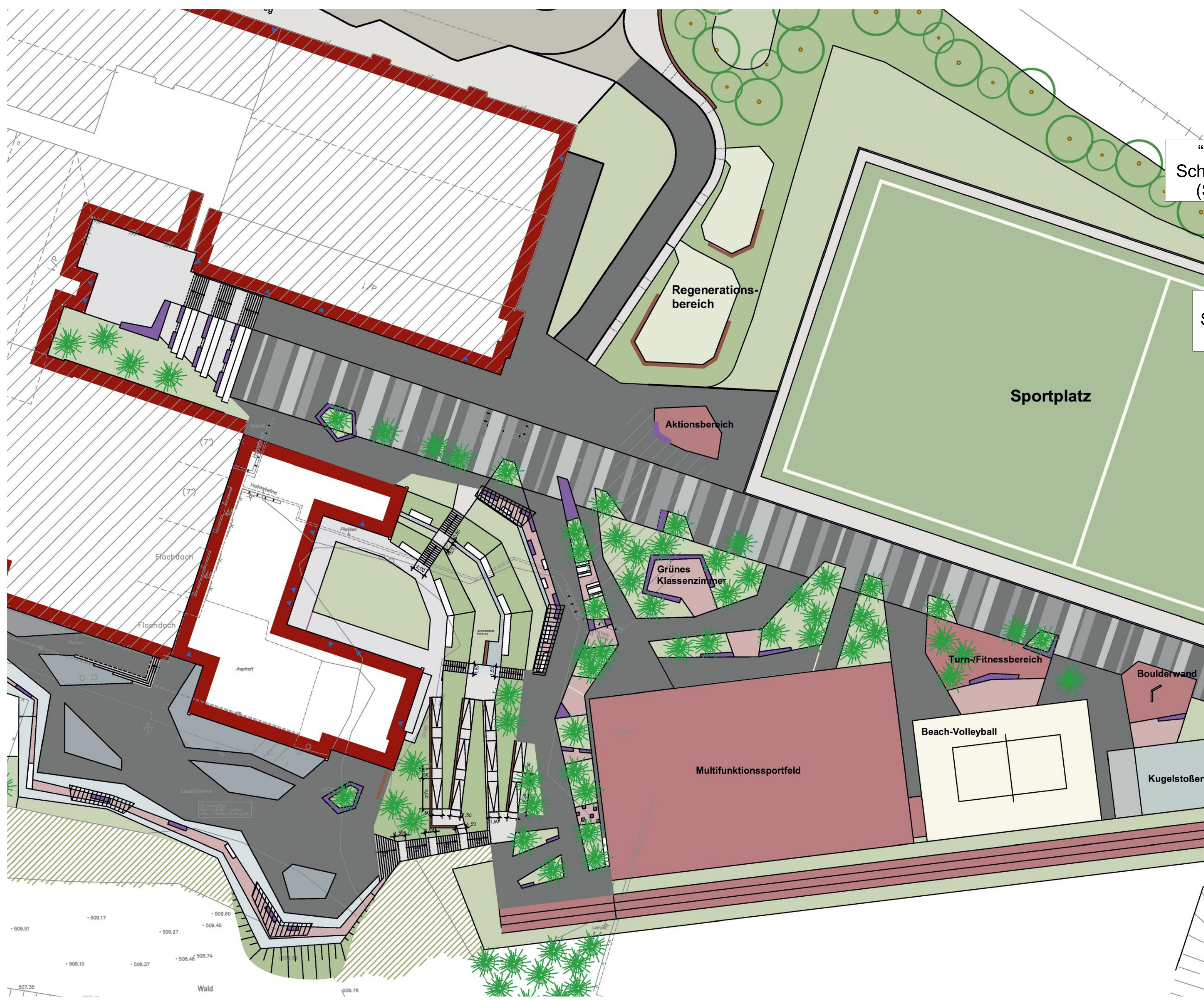
Gestaltungsplan integrative Freianlagen (Planausschnitt)
